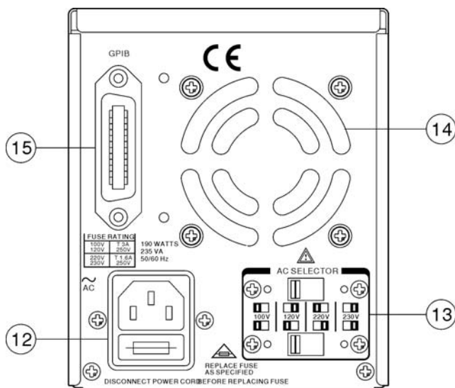
図 4-2 リアパネル
