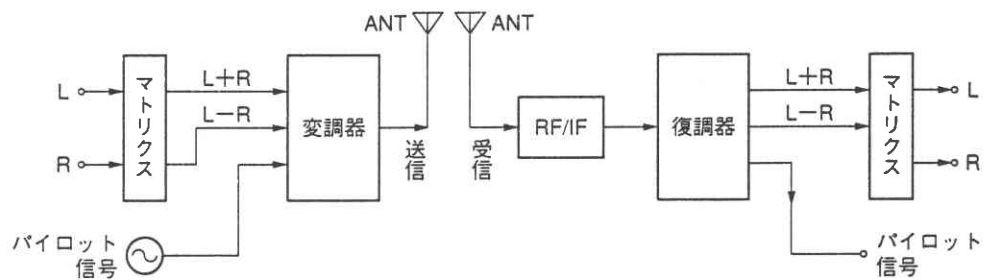
1-2図 AMステレオの基本ブロック図
