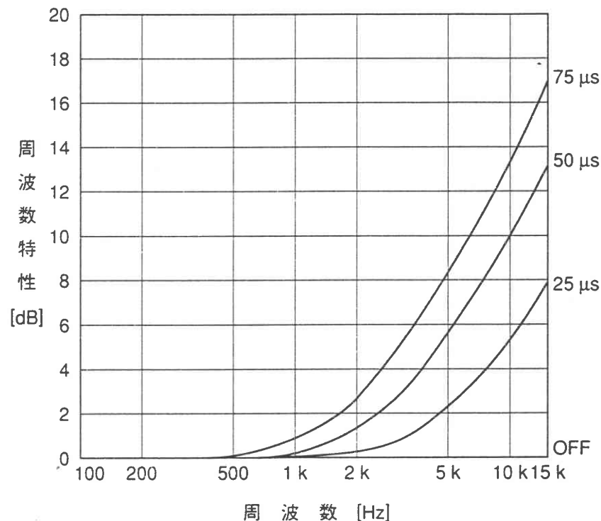
4-2図 プリエンファシス特性
