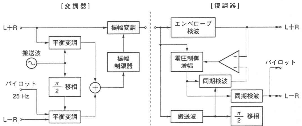
1-3図 C-QUAM方式
