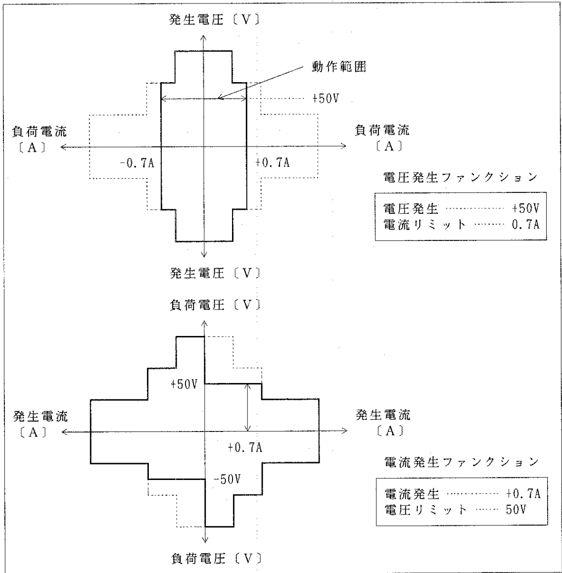
図 1 - 5 電圧、電流リミッタの設定例
