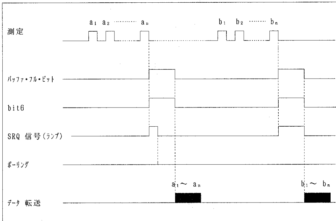
図 5 - 9 バッファ・フル・ビットのタイミング図
