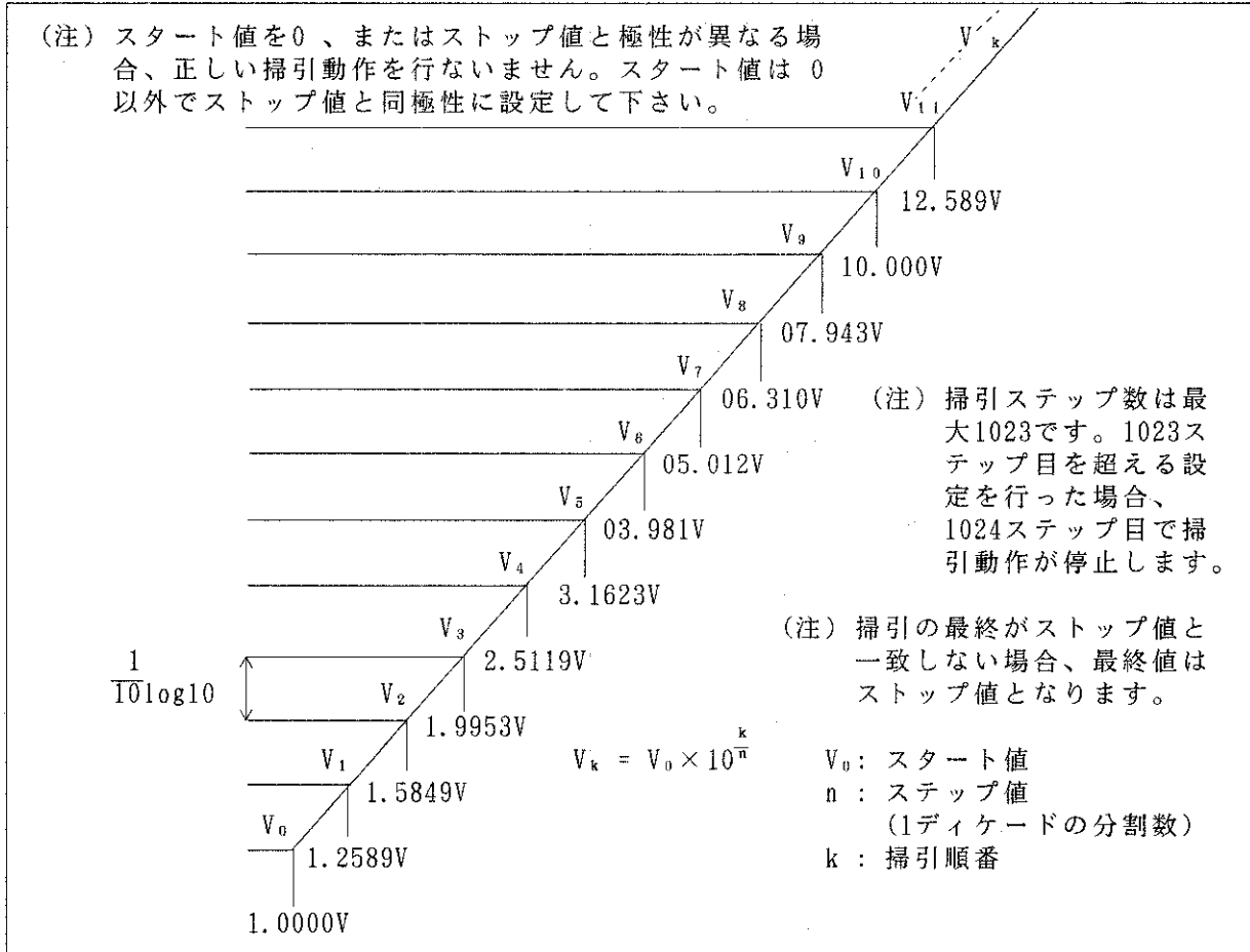
図 3 - 2 ログ掃引
