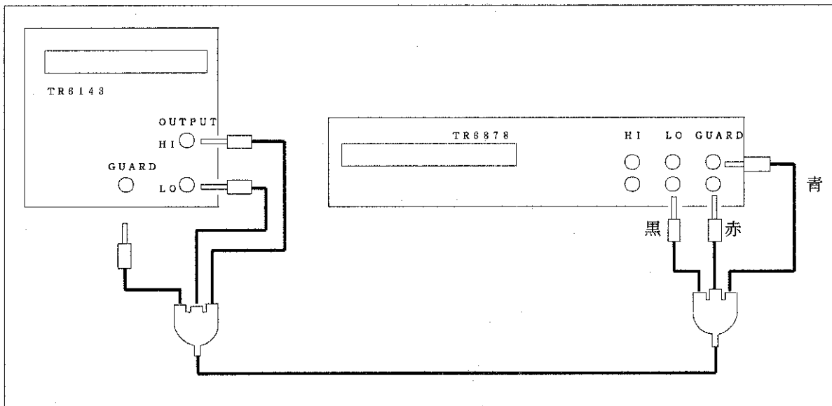
図 6 - 5 デジタル電流計との接続方法
