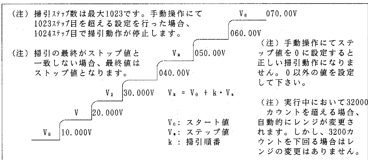
図 3 - 1 リニヤ掃引
