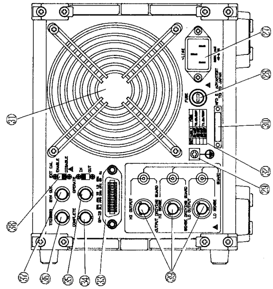
図 2-5 背面パネル
