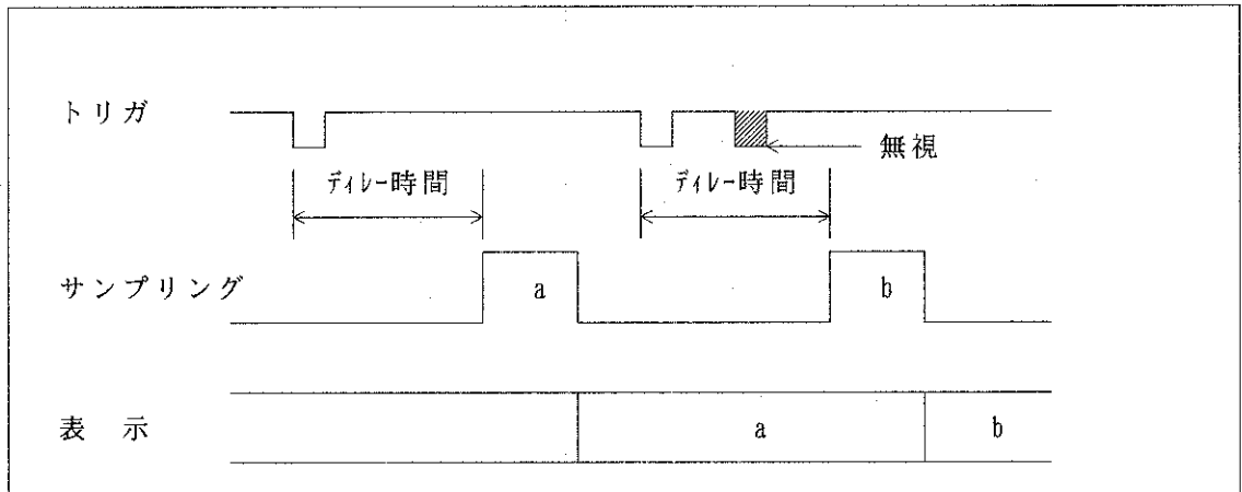
図 2 - 16 HOLD モード
