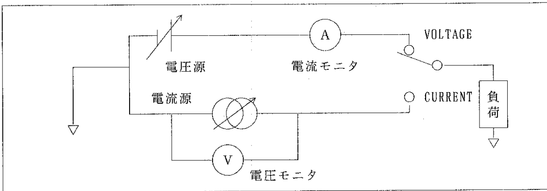
図 1 - 3 等価回路
