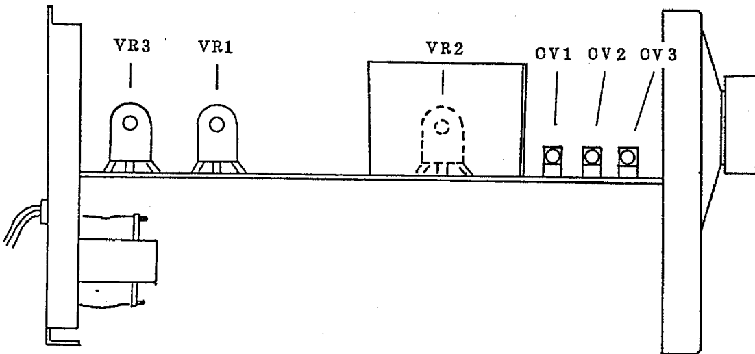
〔第5図〕 調整個所配置図
