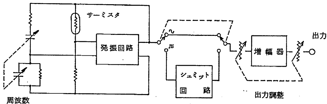
〔第3図〕 ブロックダイアグラム
